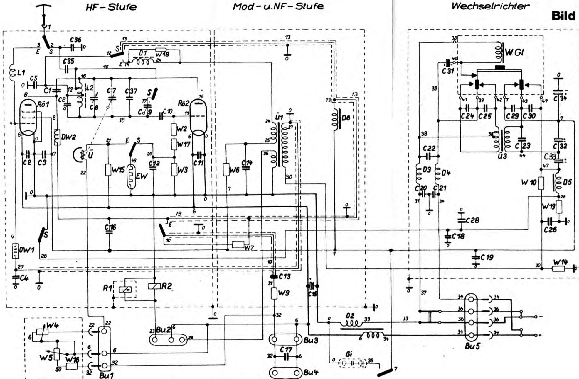
Gesamtschaltbild des Feldfunksprechers f 1
