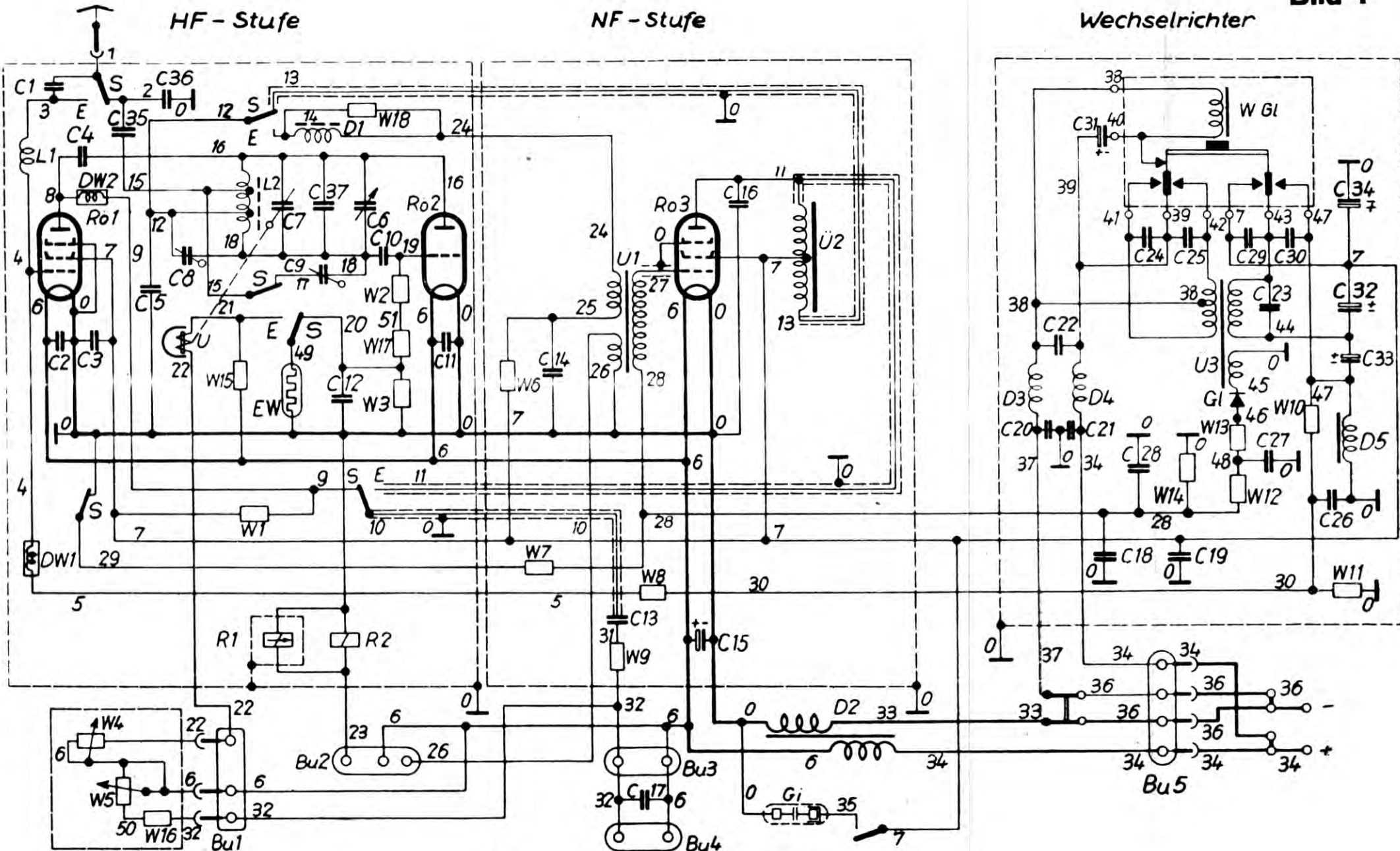
Gesamtschaltbild des Feldfunksprechers f
