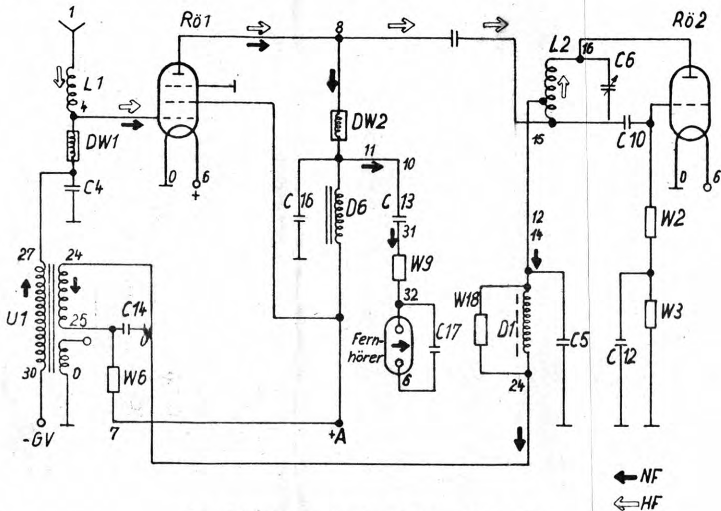
Vereinfachte Empfängerschaltung FFusp f1
