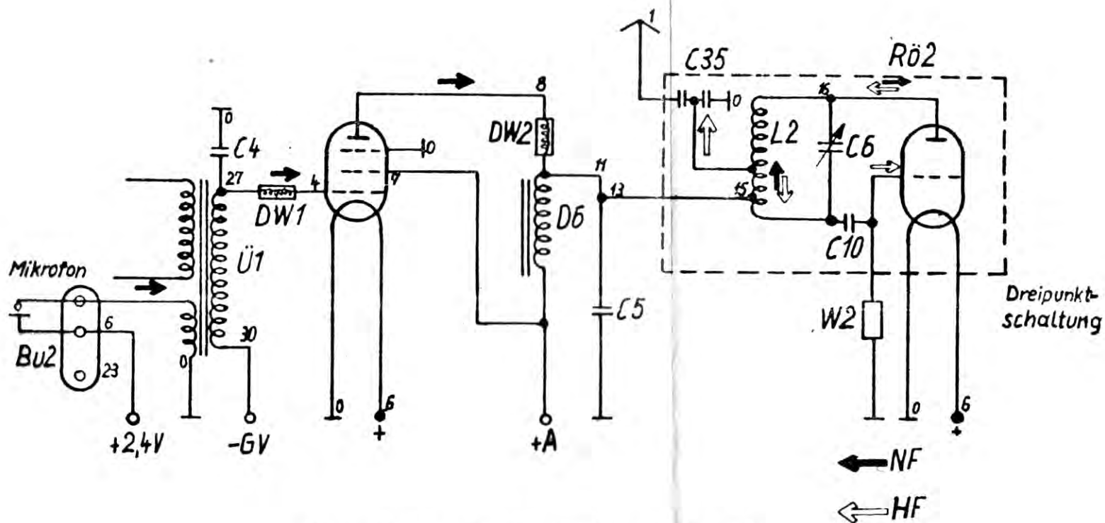
Vereinfachte Senderschaltung FFusp f1
