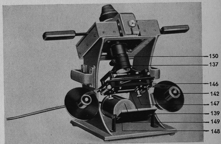
Abb. 24. Auswertegerät, Rückansicht
