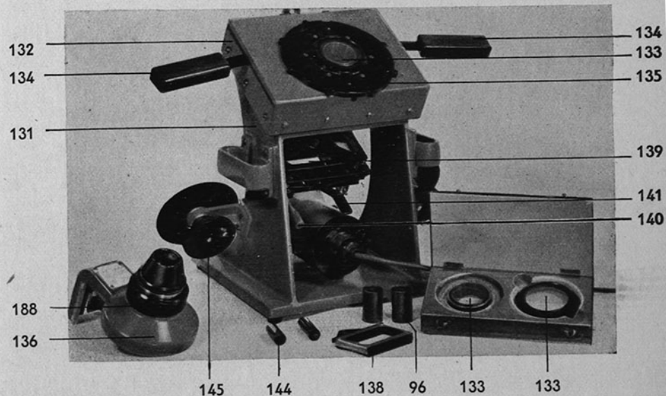
Abb. 23. Auswertegerät, Vorderansicht
